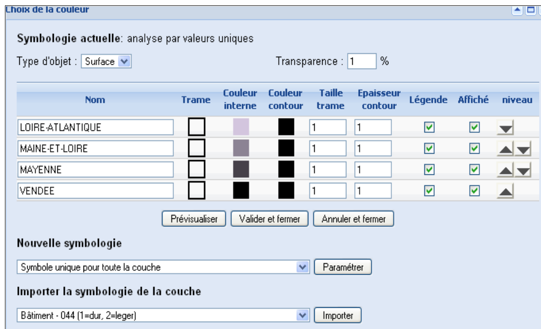
Figure 36: Fenêtre de modification de la symbologie présentant une symbologie de type valeur unique surface
